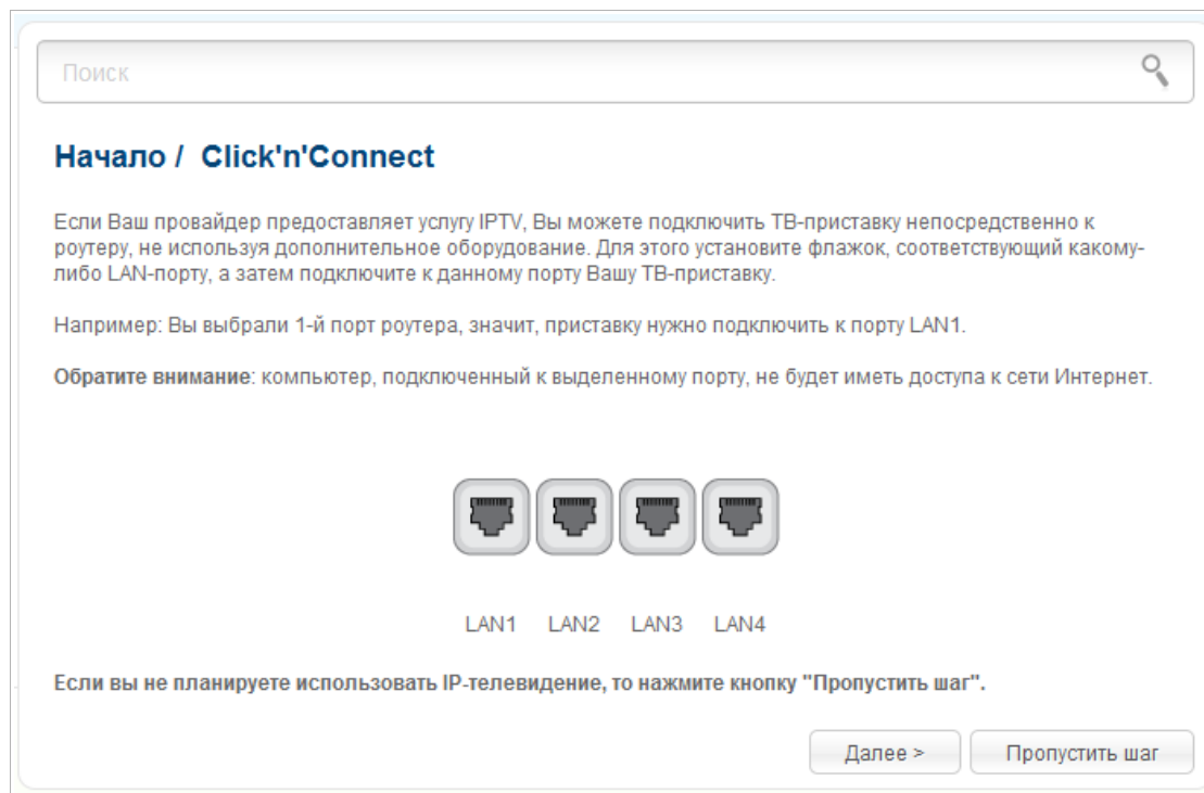
Рисунок 75. Выбор LAN-порта для подключения IPTV-приставки.
