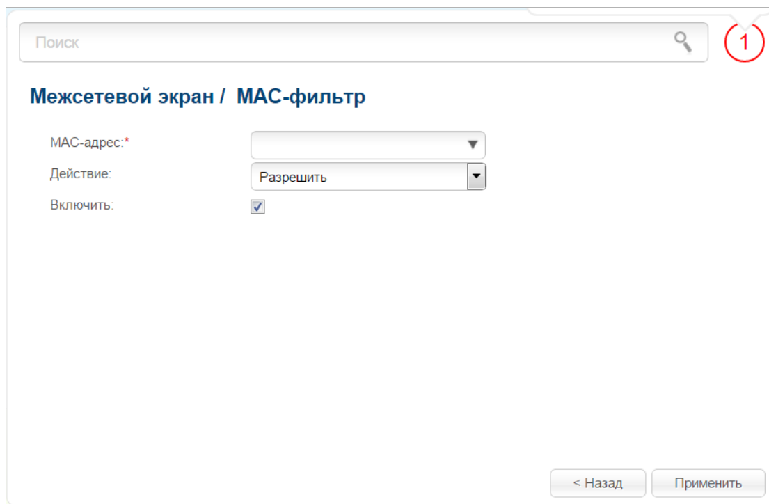
Рисунок 158. Страница добавления правила для MAC-фильтра.
