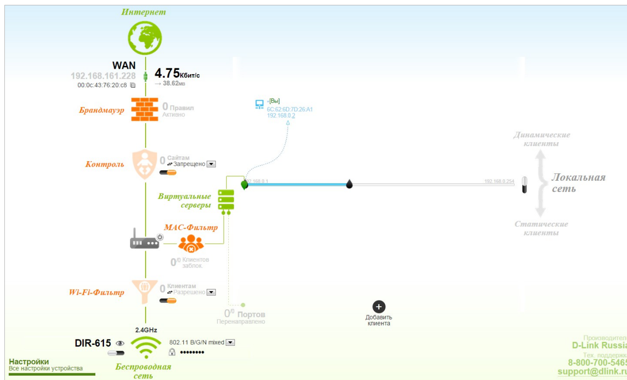
Рисунок 23. Страница Мониторинг .
