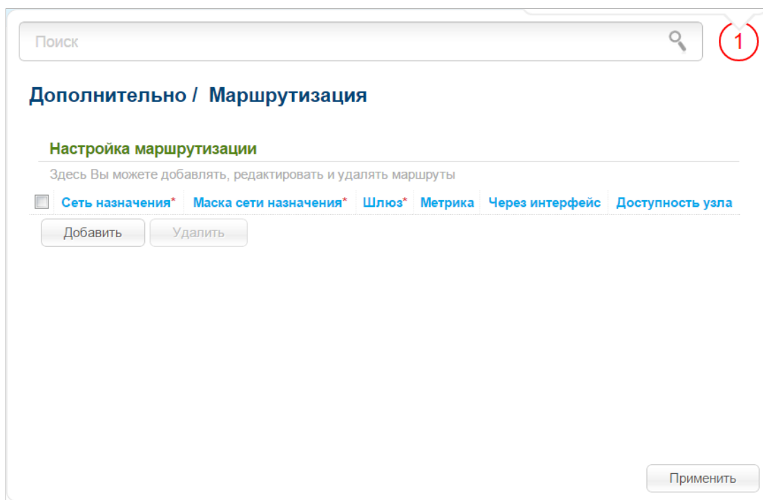
Рисунок 146. Страница Дополнительно / Маршрутизация .
