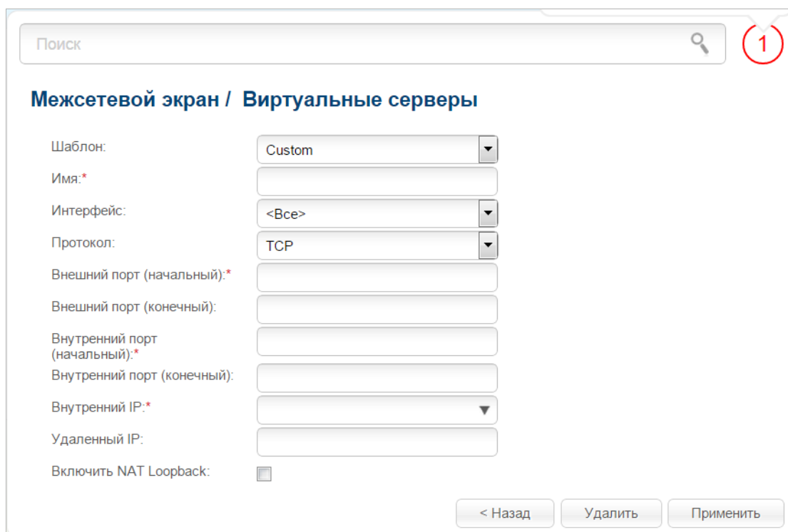
Рисунок 155. Страница добавления виртуального сервера.
